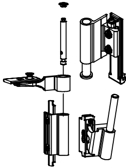
Çift açılım pencere üst menteşesi (80kg) Tilt and turn window top hinge (80kg)
