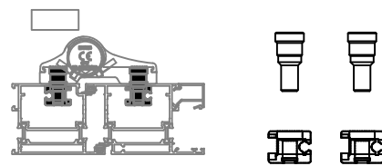
Üç yapraklı kapı menteşesi için bağlantı takımı Three-leaf hinges door for counterplates
