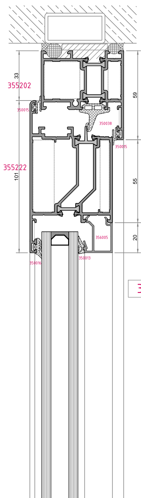
dışa açılım kapı outside opening door
