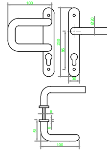
Düz-kıvrık aynalı kol Flat-curve mirrored handles
