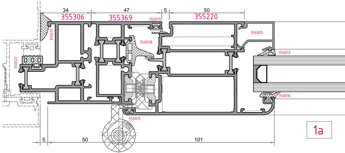
dışa açılım kapi outside opening door
