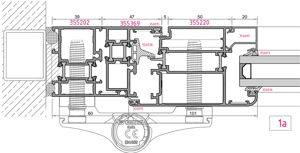
dişā acılım kapı outside opening door
